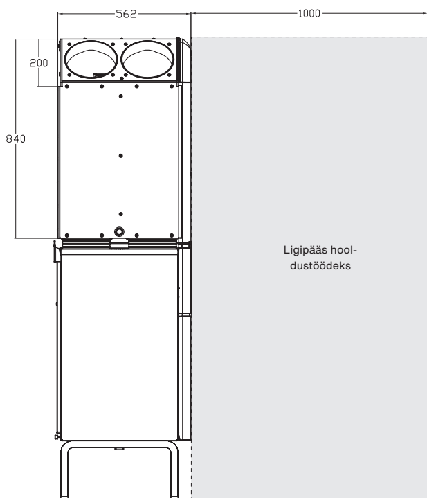
Külgvaade
