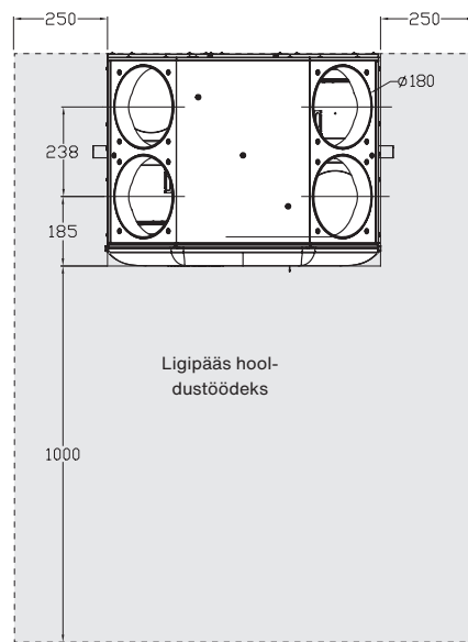
Pealtvaade
