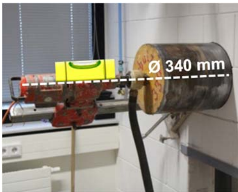
Abb. 2 Kernlochbohrung durchführen
