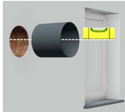
Abb. 3 Wandeinbaurohr einschieben
